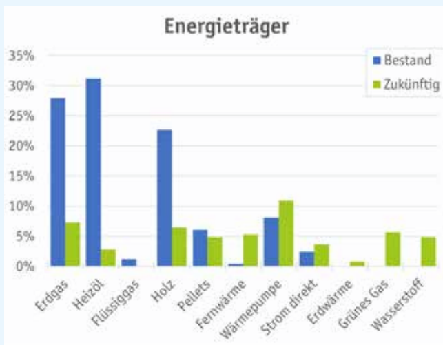
Verteilung der Energieträger für die Heizung im Bestand (blau) und zukünftig (grün).
