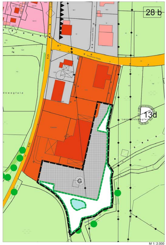
18. Änderung des Flächennutzungsplans der Stadt Feuchtwangen M 1: 2.000
